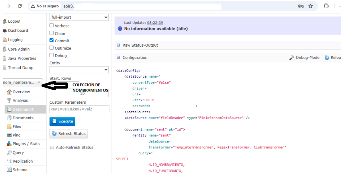
Imagen 3: Indexador SOLR con QUERY de extracción de datos desde Base de datos Oracle
